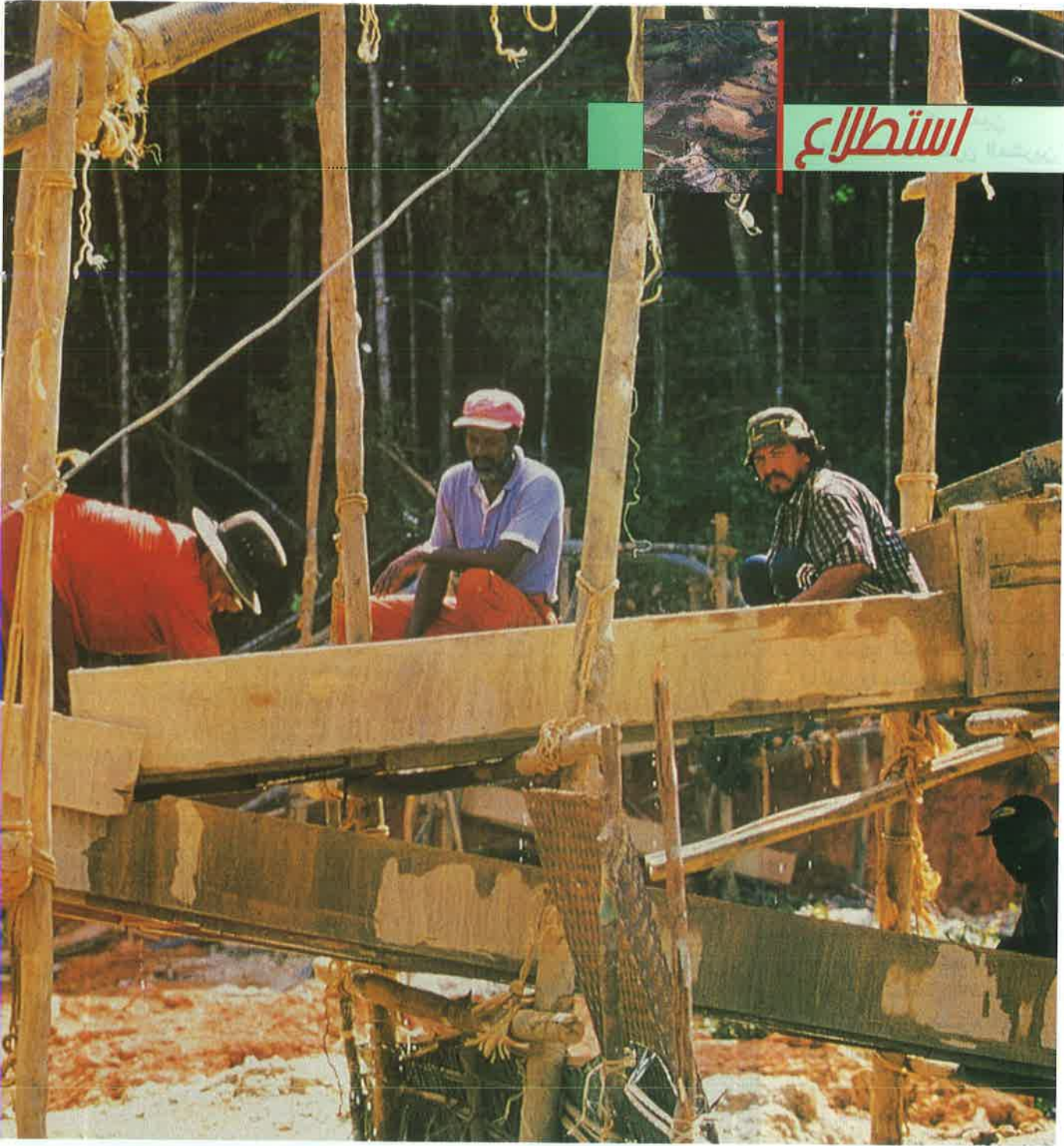
● في هذا البناء الخشبي تُغربل التربة لتصفية ذرات الذهب
